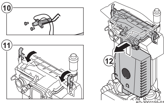
Rys.81 Kontrola
